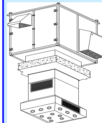
FEHU-G tetőre telepített légkezelő
