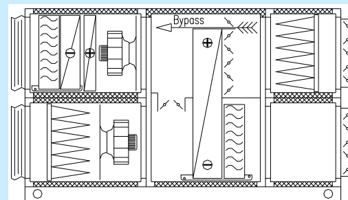
FEHU-UH uszodai építőelemes légkezelő
