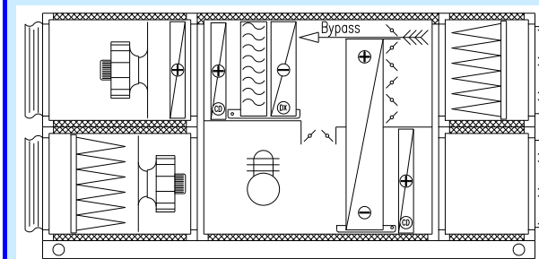
FEHU-UE uszodai építőelemes légkezelő
