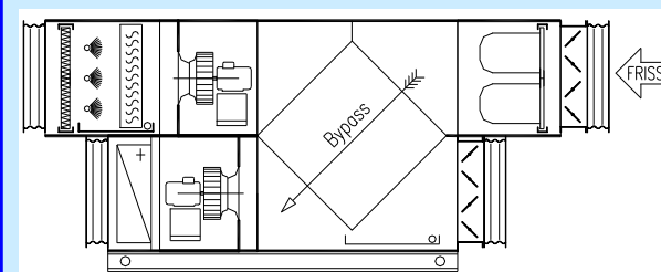
FEHU-E építőelemes légkezelő
