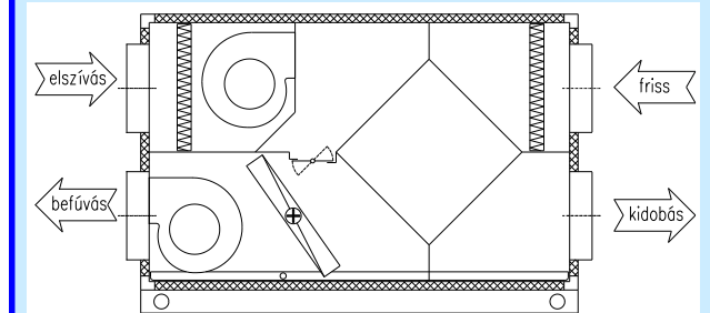
FEHU-UTV uszodai kompakt légkezelő
