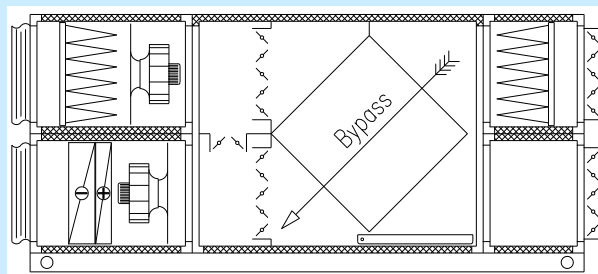
FEHU-UL uszodai építőelemes légkezelő
